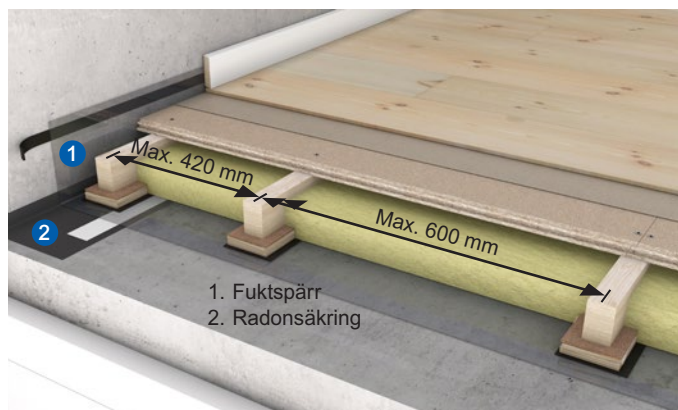
Figur 1 Undergolv på betongdäck ska alltid utföras med fuktspärr och radonsäkring på betongytan.
