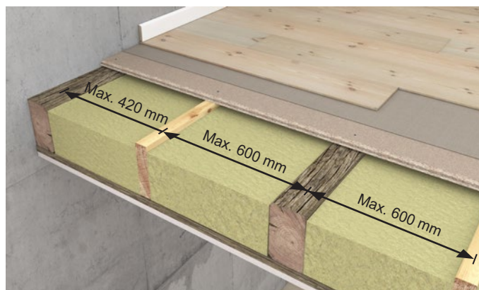
Figur 2 Äldre bjälklag med en extra balk mellan de befintliga golvbjälkarna för att minska spännvidden till max 600 mm. Alternativt kan bjälklaget förstärkas, se Faktablad #1S Förstärkning av äldre bjälklag på kronospan-se.se.
